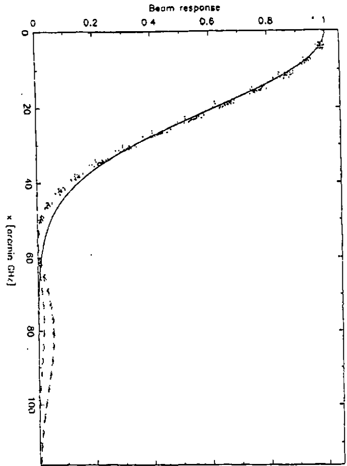
20cm gaussian fit (x=0-35)
